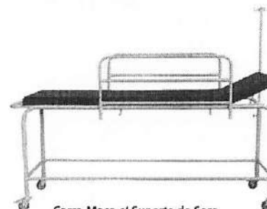
Carro Maca c/ Suporte de Soro MAC1003 Altura: 0,76m Largura: 1,62m Profundidade: 0,56m
